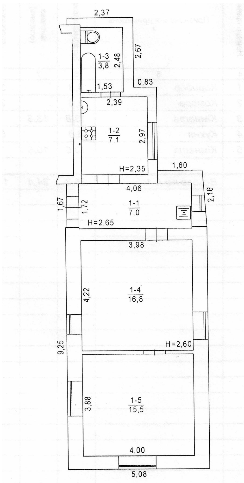
План дома В-1
